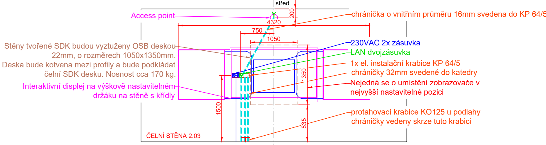
Stavební příprava pro interaktivní displej na výškově nastavitelném držáku na stěnu
